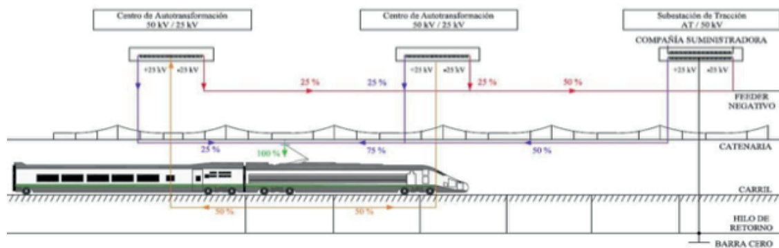
Imagen 1: Sistema eléctrico ferroviario
